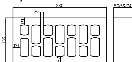
Croquis de la Pieza en mm.
