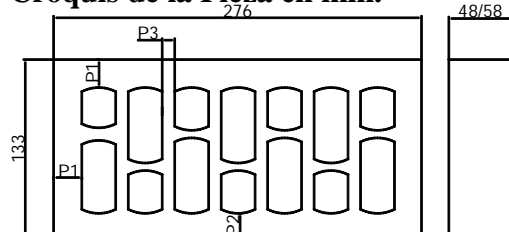
Croquis de la Pieza en mm.
