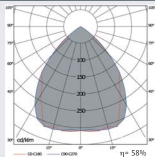
2 TC-TEL 26W
