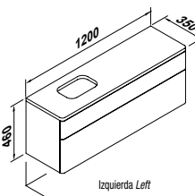
MUEBLE BASE DE 120 x 35 cm. 120 / 35 cm. VANITY UNIT
