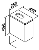
MUEBLE BASE LAVAMANOS 25 x 45 # 3817177 (Aqua) / # 3817176 (Antracita) 25 x 45 HANDBASIN VANITY UNIT
