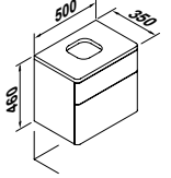
MUEBLE BASE LAVAMANOS 50 X 35 cm. # 3817277 (Aqua) / # 3817276 (Antracita) 50 x 35 cm. HANDBASIN VANITY UNIT
