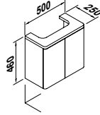
MUEBLE BASE LAVAMANOS 50 x 25 # 3817077 (Aqua) / # 3817076 (Antracita) 50 x 25 HANDBASIN VANITY UNIT
