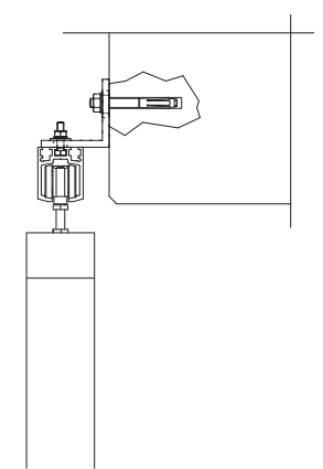
Front-fixation
