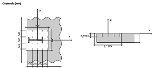
Detalle del apoyo de rampa. Consideraciones previas.
