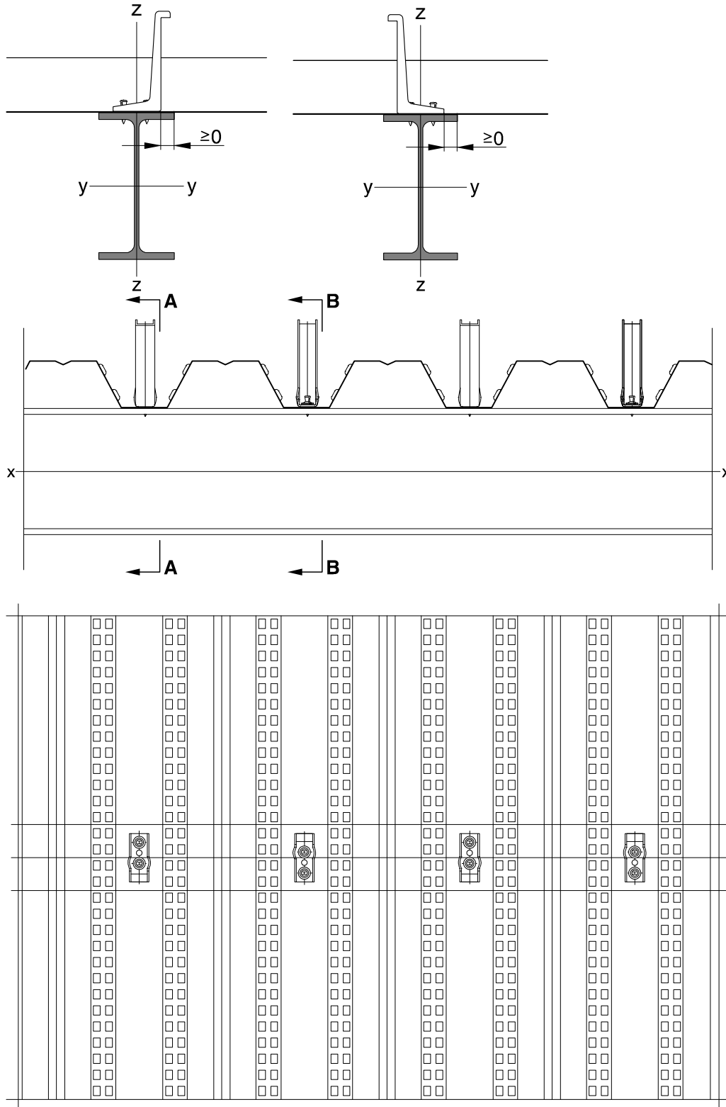
Sección B-B:
