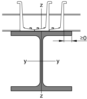
Sección B-B:
