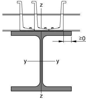
Sección A-A:
