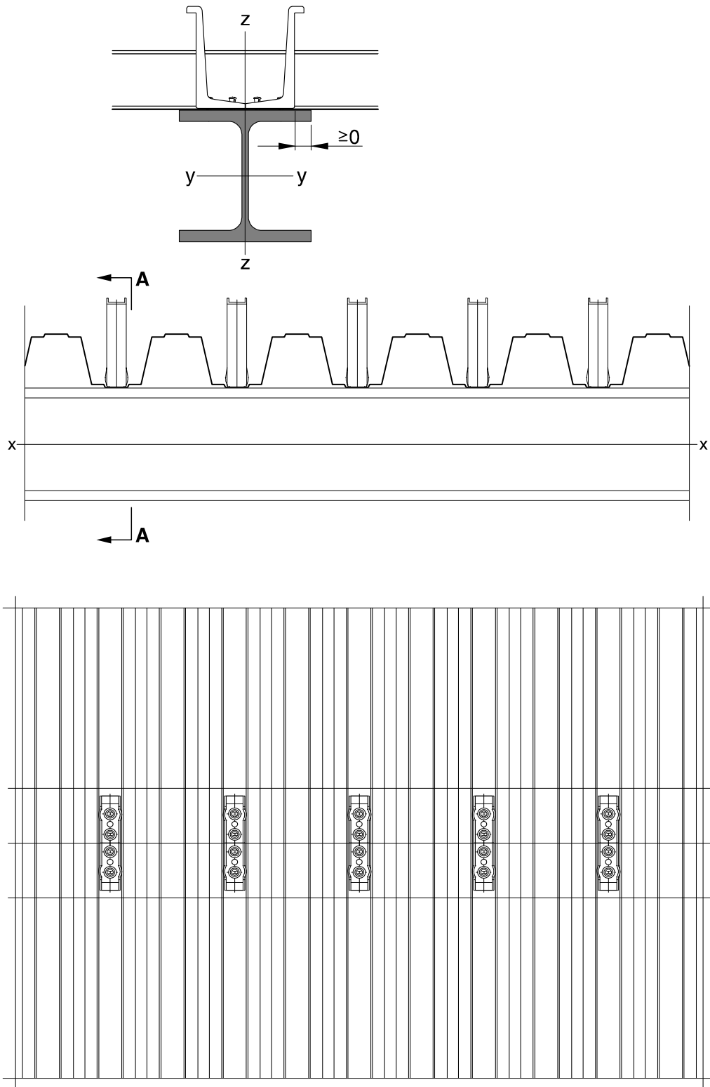
Sección A-A:
