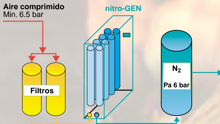
Diagrama baja presión
