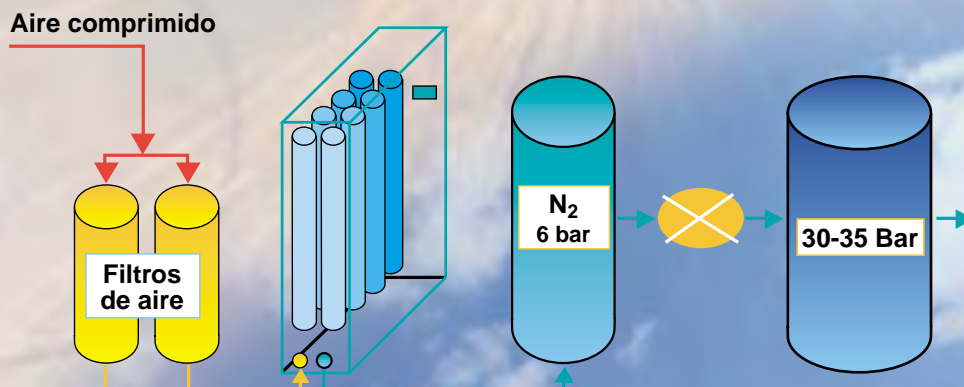
Diagrama alta presión
