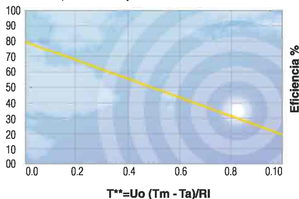
* Curva correspondiente a ensayo TÜV
