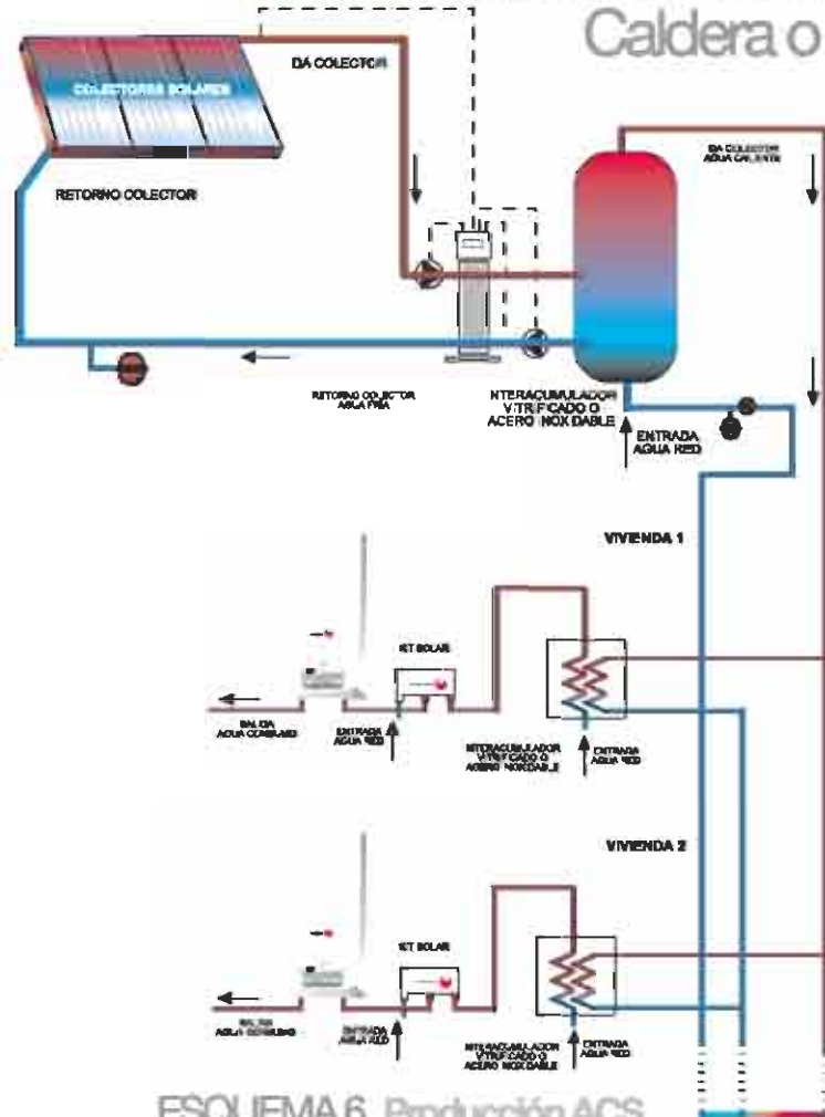
ESQUEMA 6. Producción ACS
