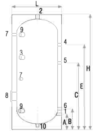
Esquema de conexiones BDH 1500
