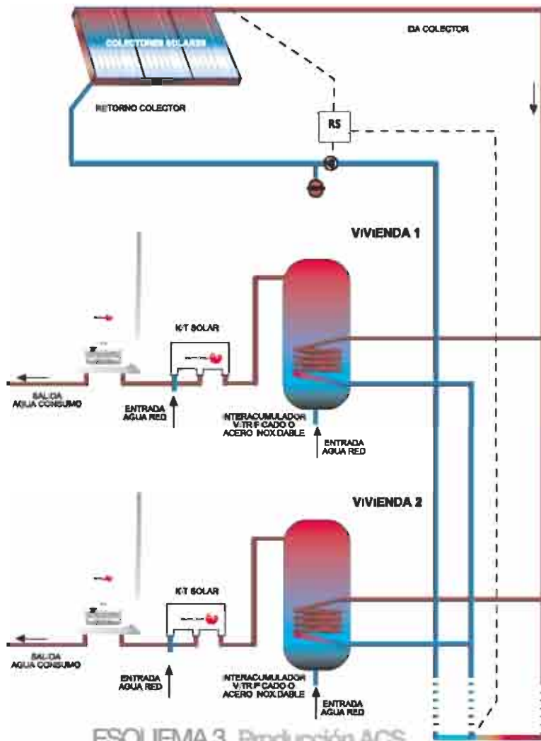
ESQUEMA 3. Producción ACS
