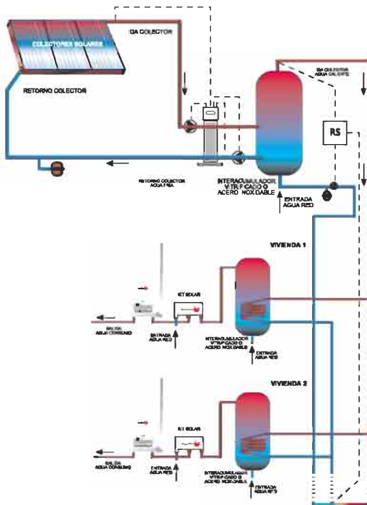
ESQUEMA 5. Producción ACS
