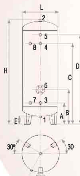
Esquema de conexiones BDC 750
