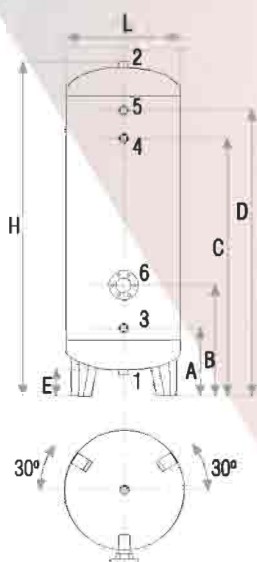
Esquema de conexiones BDC 500
