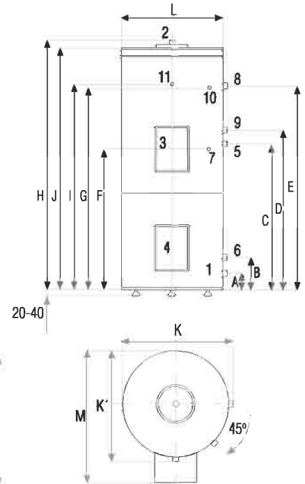
Esquema de conexiones BDS 1200 - 2200-1300-2300
