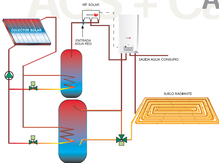
Esquema 1. Distribución de energía en primario.
