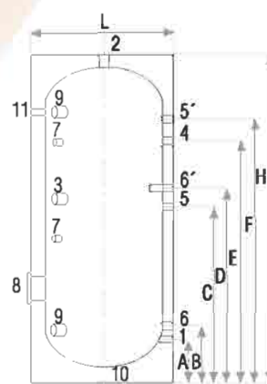
Esquema de conexiones BDH 2500
