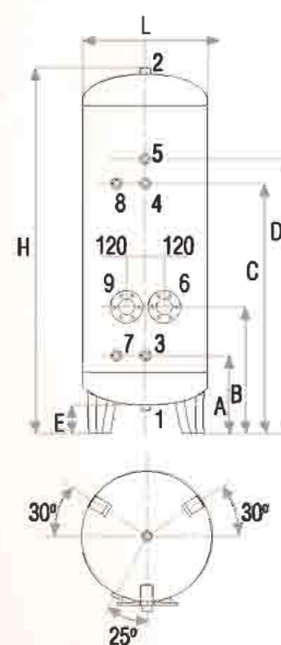
Esquema de conexiones BDC 1000-1500-2000
