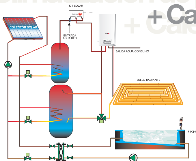
Esquema 1. Distribución de energía en primario.
