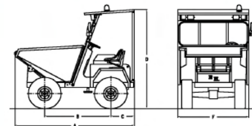
Dimensiones (mm) / Dimensions (mm)
