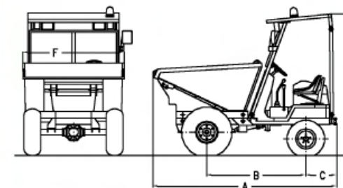
Dimensiones (mm) / Dimensions (mm)
