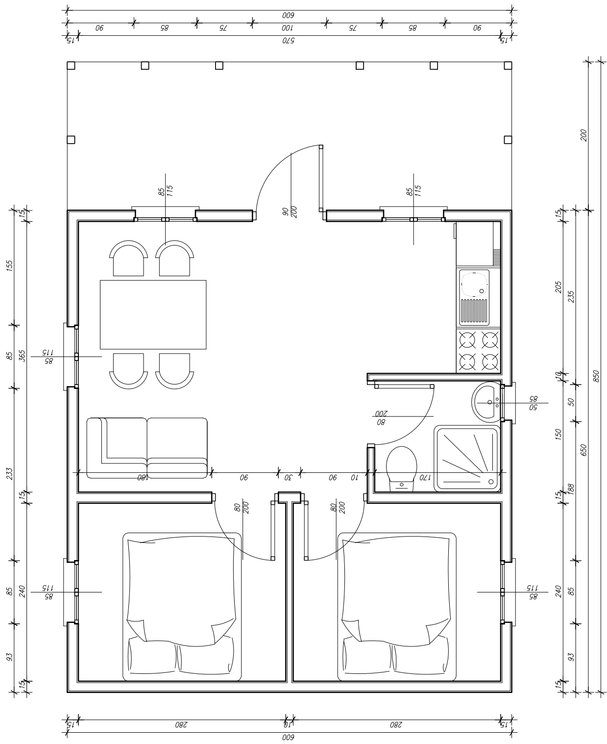
RZUT PARTERU SKALA 1:50
