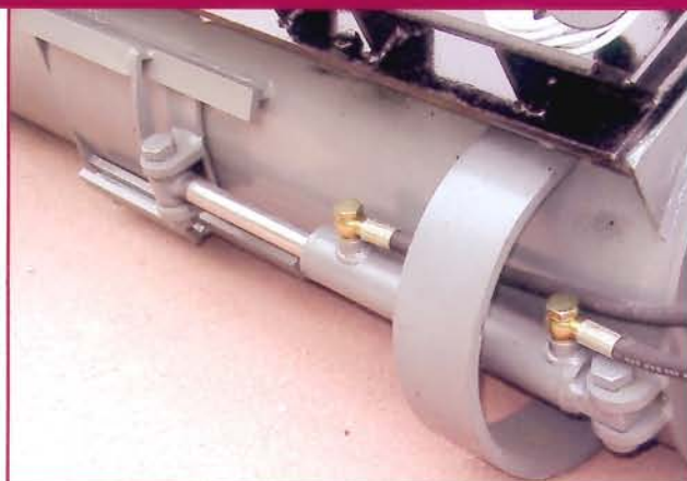
▲ Sistema de vaciado Discharging system
