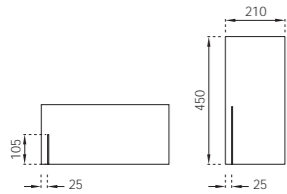
Señal rectangular alta Rectangular high sign
