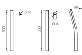
Soporte para señal baja Support for low sign
