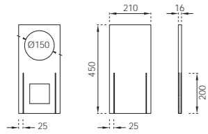
Señal rectangular baja Rectangular low sign
