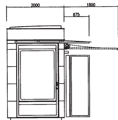
ALZADO LATERAL
