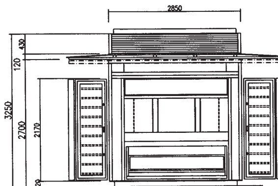
ALZADO FRONTAL
