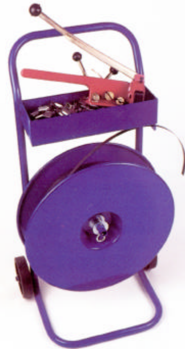
Carro portabobinas
