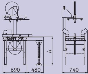
ALTURA PLANO DE TRABAJO MÁX./MIN.
