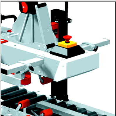
Guía de presión lateral y paro de emergencia en la zona central
