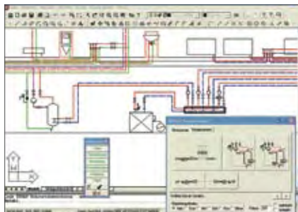
RAUCAD - esquema de la red de tubos
