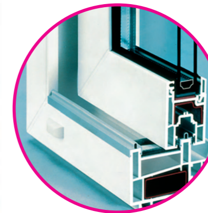
Perfil de ventana REHAU-S717
