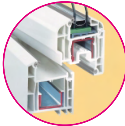
Perfil de diseño redondeado
