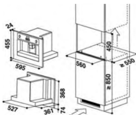
ESQUEMA DE INSTALACIÓN ACE-100
