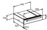
ESQUEMA DE INSTALACIÓN WD-140
