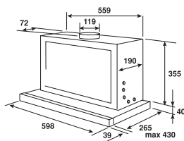
ESQUEMA DE INSTALACIÓN AKR-633 GY-2
