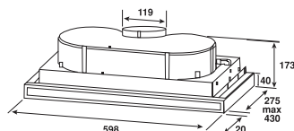
ESQUEMA DE INSTALACIÓN AKR-665
