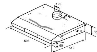
ESQUEMA DE INSTALACIÓN AKR-409
