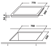
ESQUEMA DE INSTALACIÓN AKM-972
