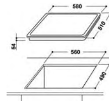
ESQUEMA DE INSTALACIÓN ACM-703 AKM-980 ACM-701
