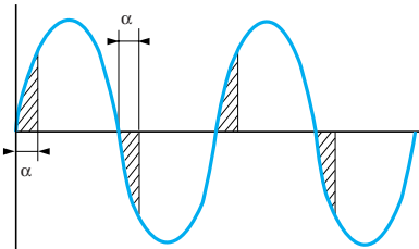
Ángulo de cebado
