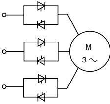
Esquema de principio
