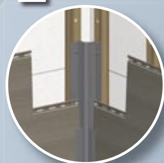
Perfil de esquina interior 2
