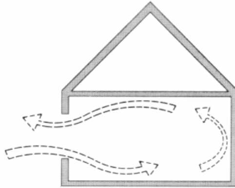
Figura 12: ventilación producida por diferencias de temperatura.
