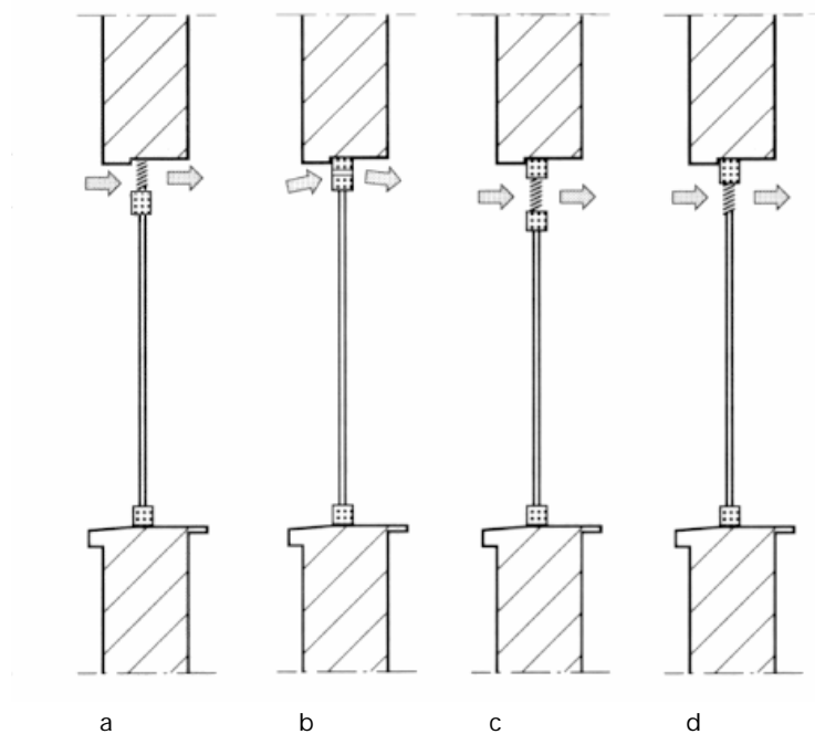
Figura 11 : diferentes posiciones de los mecanismos para ventilación en las ventanas.
