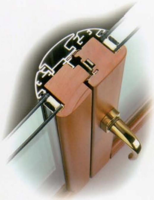
Sección carpintería mixta. Piel aluminio exterior, madera al interior
