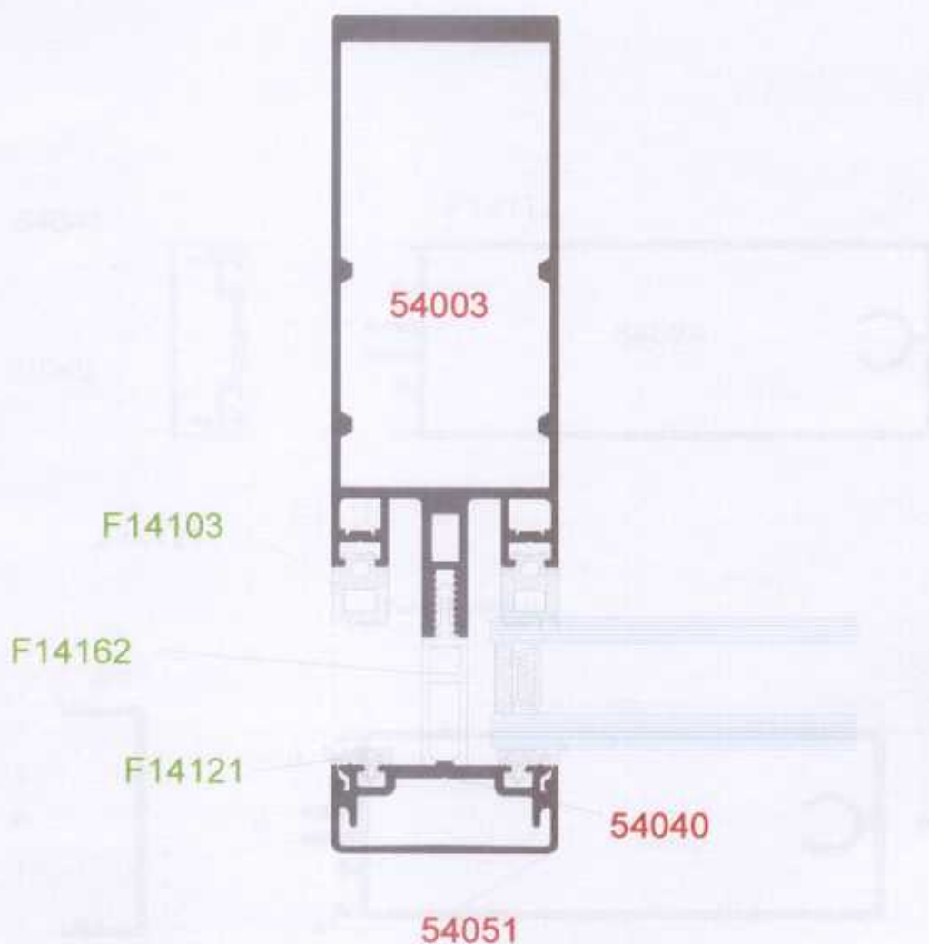
Sección Horizontal
