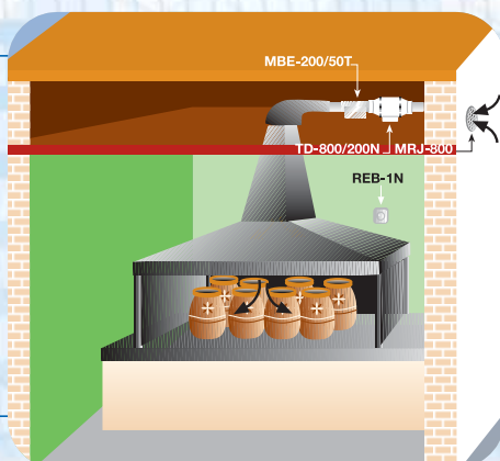
Tunel de cerámica
