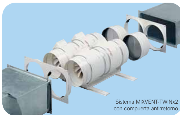
Sistema MIXVENT-TWINx2
