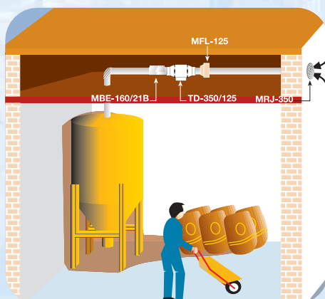
Tolva de frutos secos
