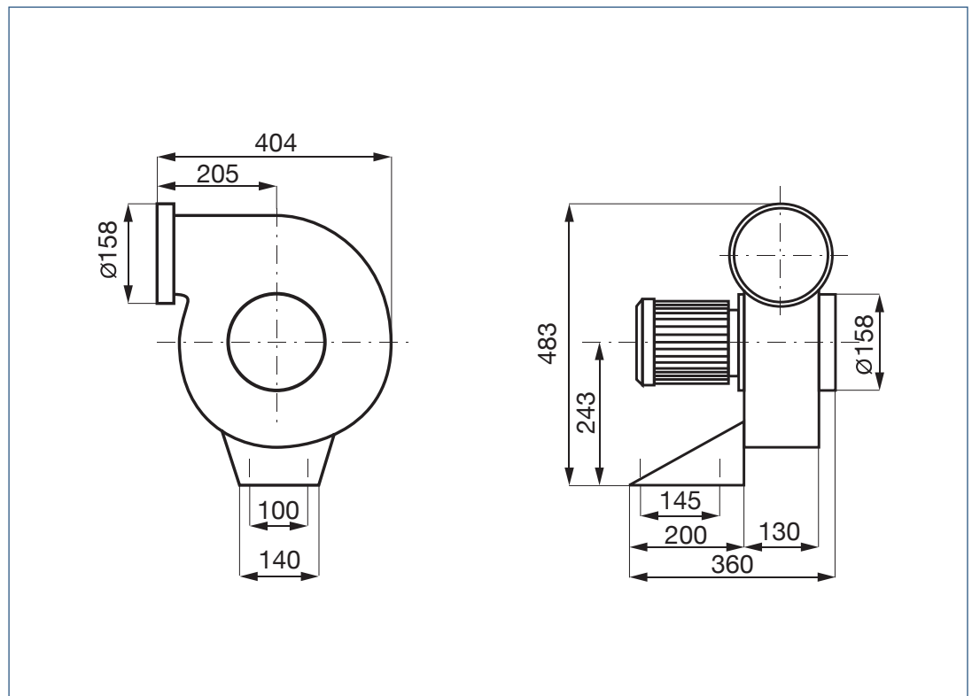
DIMENSIONES (mm)
