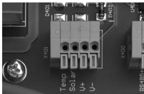
(Fig.) Bloque de conexión para el sensor de radiación
