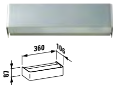
Aplique mural, aluminio. 4.9602.1.080.007.1
