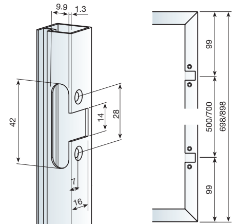
MECANIZADO Y SITUACIÓN DE LAS BISAGRAS
