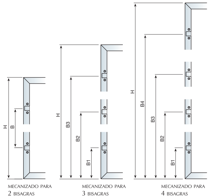
MECANIZADO Y SITUACIÓN DE LAS BISAGRAS
