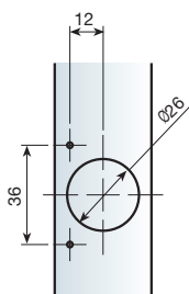
MECANIZADO Y SITUACIÓN DE LAS BISAGRAS
