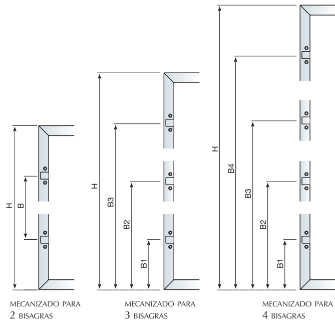
MECANIZADO Y SITUACIÓN DE LAS BISAGRAS
