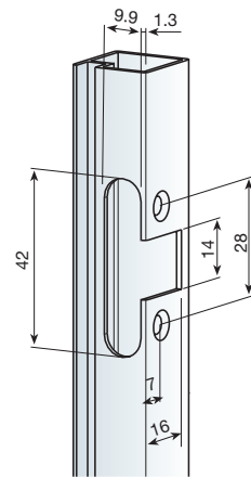
MECANIZADO Y SITUACIÓN DE LAS BISAGRAS
