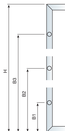
MECANIZADO PARA 3 BISAGRAS
