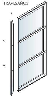
MONTAJE DE LAS PUERTAS CON TRAVESAÑOS
