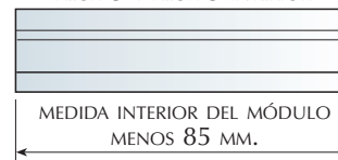
CÁLCULO DEL FONDO PARA CAJONES ALUX-3 Y ALUX-3 INTERIOR
