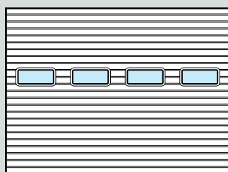
Con ventana seccional tipo A Medida libre: 635 x 245 mm Alto panel: 500 mm
