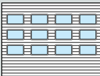
Con ventana sándwich tipo E Medida libre: 725 x 370 mm Para Alto panel: 625, 750 mm
