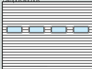
Con ventana sándwich tipo A Medida libre: 635 x 245 mm Para Alto panel: 625, 750 mm
