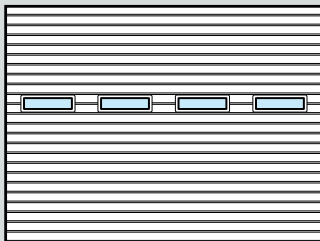
Con ventana sándwich tipo D Medida libre: 602 x 132 mm Para Alto panel: 625, 750 mm
