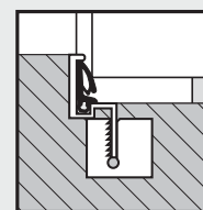
Perfil de tope con junta (sólo en puertas con aislamiento acústico)
