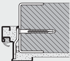
Cerco angular Montaje soldado
