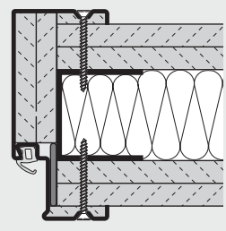
Instalación en topes de tabique prefabricado de acero (no para HG19)
