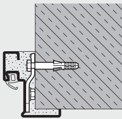
Cerco angular Montaje por tacos (no para HG19)
