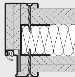
Cerco angular y cerco complementario o cerco integral para yeso encartonado GKF, montaje atornillado
