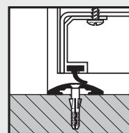
Perfil inferior de aluminio con junta, cerco con galga umbral
