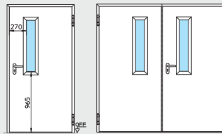
Acristamiento fig. 1
