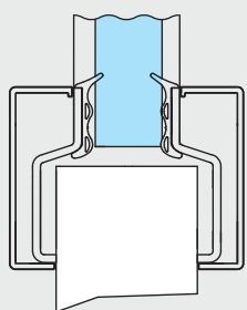
Perfil de recubrimiento de aluminio
