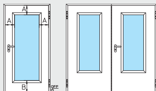
Acristalamiento fig. 3
