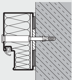
Cerco de bloque montaje por tacos cubierto (no para HG19)
