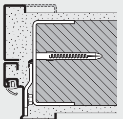
Cerco angular y cerco complementario Montaje soldado
