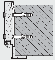
Cerco integral Montaje por tacos a través del intradós del cerco (no para HG19)
