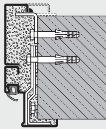
Cerco angular y cerco complementario Montaje por tacos cubierto (no para HG19)
