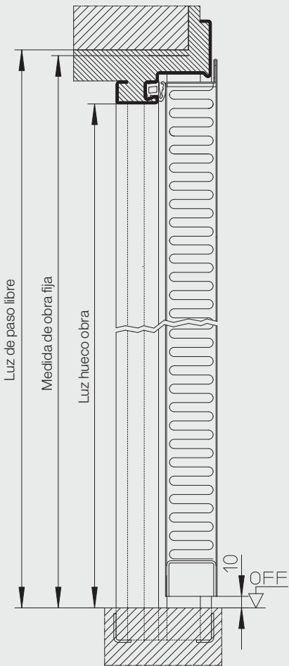
Sección vertical
