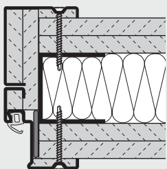
Cerco angular y cerco complementario o cerco integral para yeso encartonado GKF, montaje atornillado El revestimiento del cerco se puede realizar, a elección, con tiras de lana mineral o de yeso encartonado
