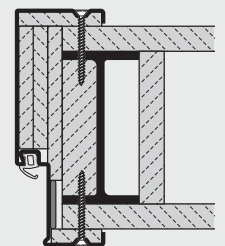
Cerco angular y cerco complementario o cerco integral para yeso encartonado GKF, montaje atornillado
