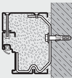
Cerco angular/de bloque Montaje por tacos (sólo para HG19)
