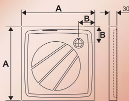
PERSEUS PRO 80 A = 800 mm PERSEUS PRO 90 A = 900 mm PERSEUS PRO 100 A = 1000 mm B = 200 mm
