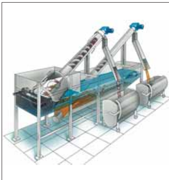
Esquema de una planta compacta ROTAMAT® Ro 5
