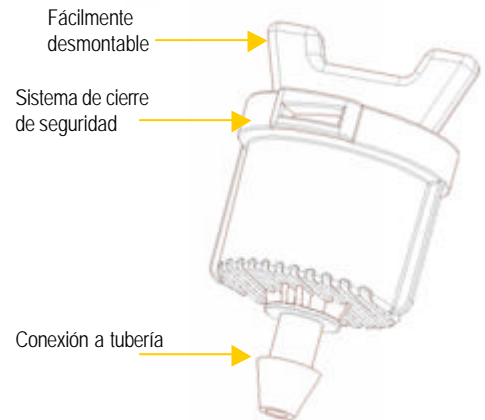
S-50-L Gotero pinchado interlinea
