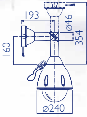
Pendant Mount 90003
