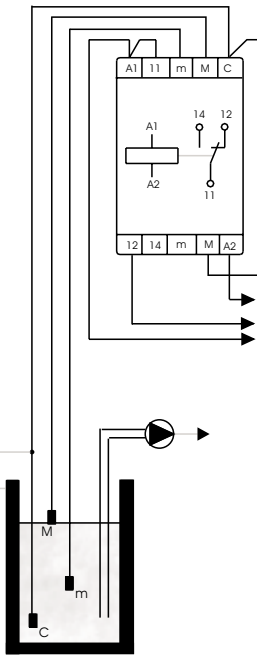
FUNCION VACIADO. DRAINING FUNCTION. Contacto (11-12)
