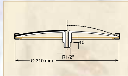
DIMENSIONES DE ROEFLEX
