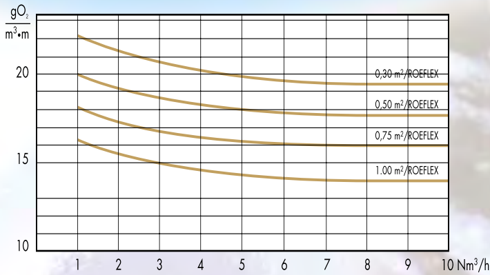
Transferencia específica de oxígeno ( g O_2/m^3 \cdot m ) en función del caudal de aire ( Nm^3/h ) y de la densidad de difusores ( m^2/ROEFLEX )
