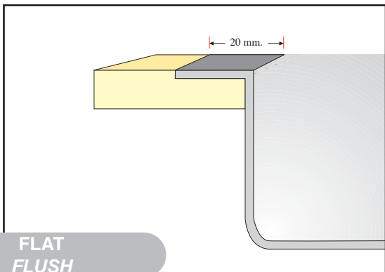
ENCASTRADO/FLAT INSET
