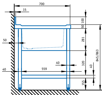
Fregadero, bastidor y estante 700
