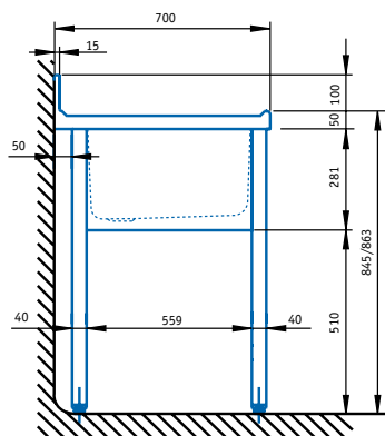
Fregadero y bastidor 700
