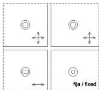
Situación de las arandelas según la posición del vidrio Washer situation depending on the glass position
