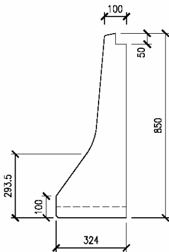
VISTA DE ALZADO (MEDIA BARRERA)
