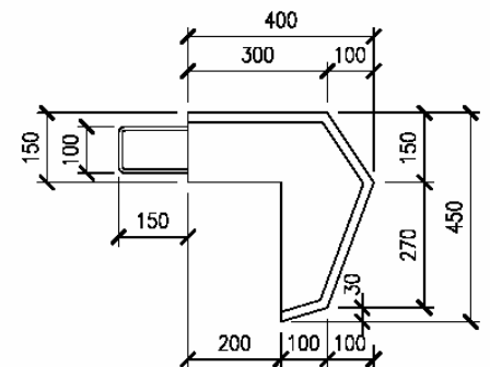
PERFIL
