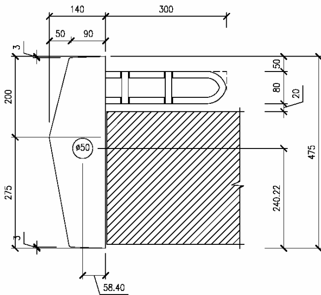
SECCION TIPO
