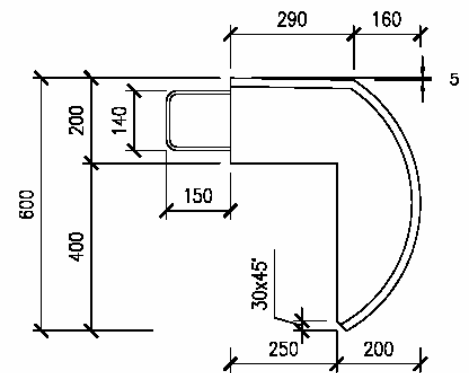
PERFIL
