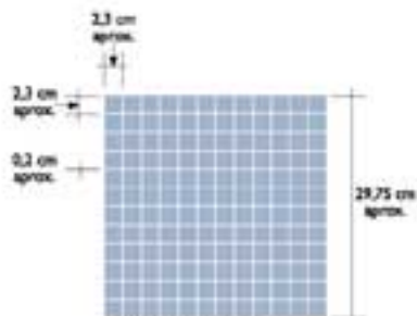
precisión 2,5x2,5 12"x12" - 30x30 cm (29,75x29,75 cm)
