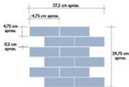
trabado síf 12"x15" - 30x37,5 cm (29,75x37,5 cm)
