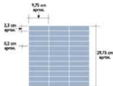
precisión 2,5x10 12"x12" - 30x30 cm (29,75x29,75 cm)
