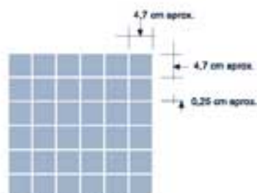
Preincisión 5x5 cm 12"x12" 30x30 cm (29,75x29,75 cm)
